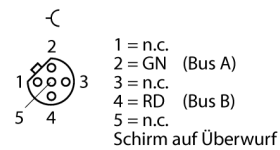
Anschlussbelegung links
