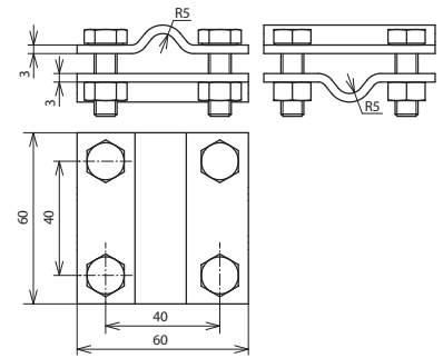
Maßbild KS 8.10 8.10 FL30 V4A
