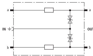
Prinzipschaltbild DRL RE 60
