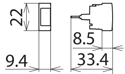
Maßbild DRL RE 60
