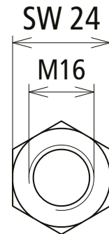
Maßbild
