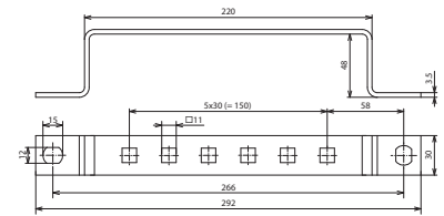
Maßbild ES 6AP 11X11 V2A
