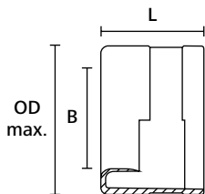
HelaGuard Endverschluss
