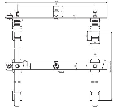
Maßbild
