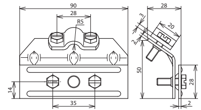
Maßbild SGK ZS 7.10 KB3.13 STTZN
