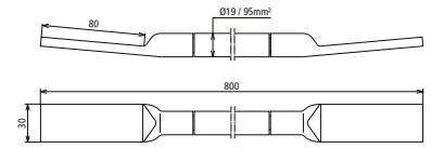
Maßbild D BEB 10 - L800 / EBS 15-03-19
