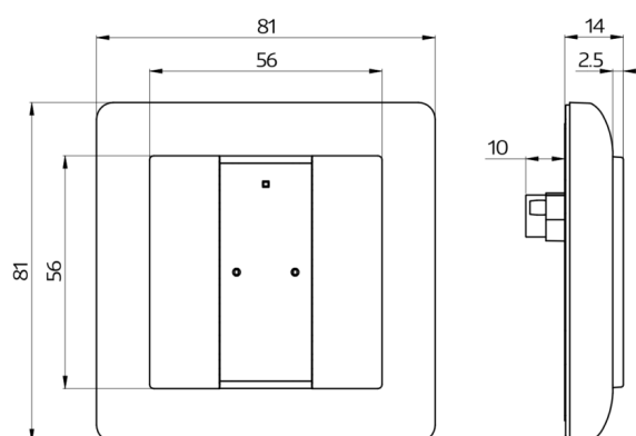
Bemaßung 93172
