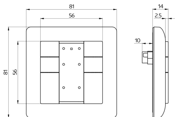
Bemaßung 93176
