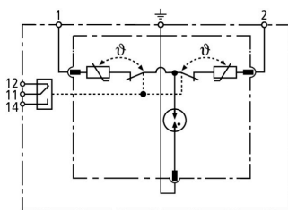
Prinzip Schaltbild DR M 2P 255 SN1803FM
