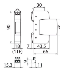
Maßbild DR M 2P 255 SN1803FM
