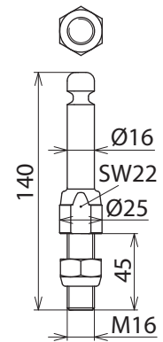
Maßbild EFP 16 RN M16 45 SSM
