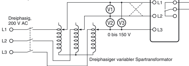
Anschlussplan 1
