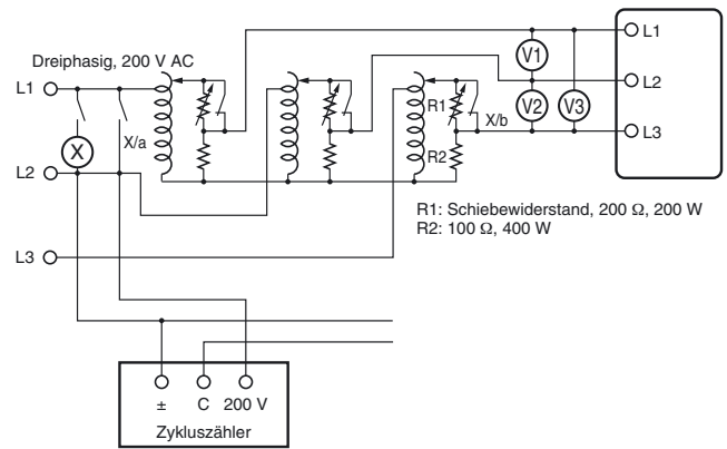
Anschlussplan 2
