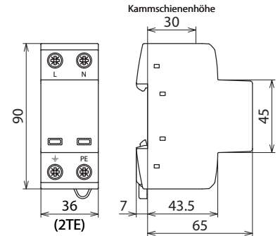
Maßbild DSH TT 2P 255
