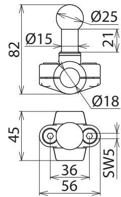
Maßbild KFP 25 RL 18
