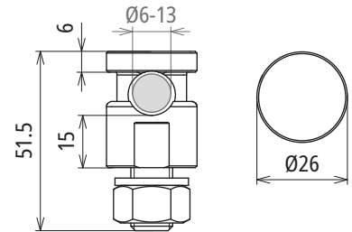
Maßbild KSV 200 13 FER V2A
