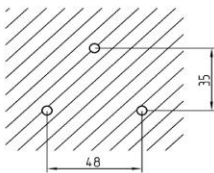
Bohrbild
