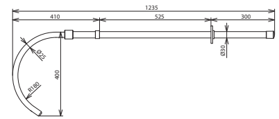
Maßbild RST 36 1000
