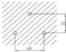
Bohrbild
