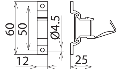
Maßbild SH 18X3 K
