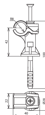
Maßbild
