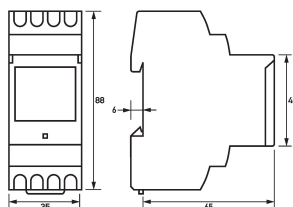
Maßzeichnung Gruppenansicht
