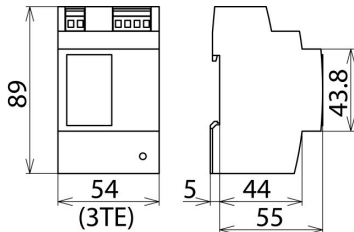
Maßbild PSU DC24 30W
