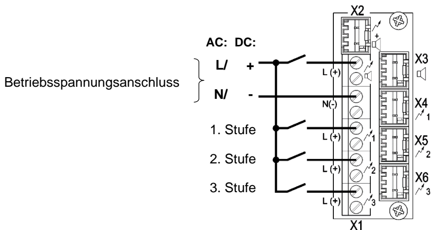
Anschlussklemme (X1)
