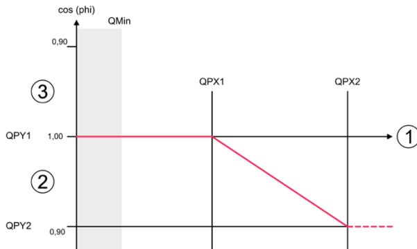
Abbildung 10: Q(P)-Kennlinie
