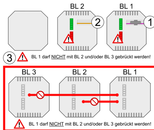
Abbildung 7: Batterielader 1 und 2 Rückseite
