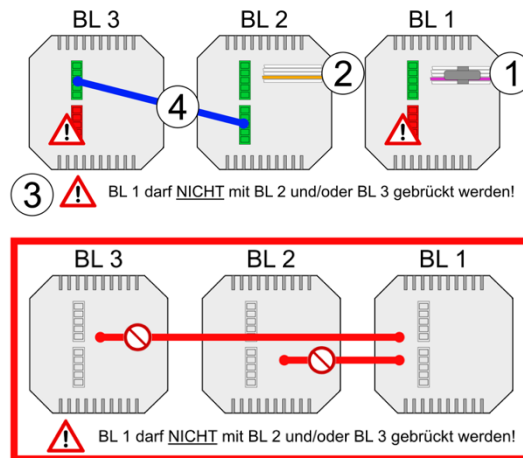
Abbildung 9: Batterielader 1, 2 und 3 Rückseite
