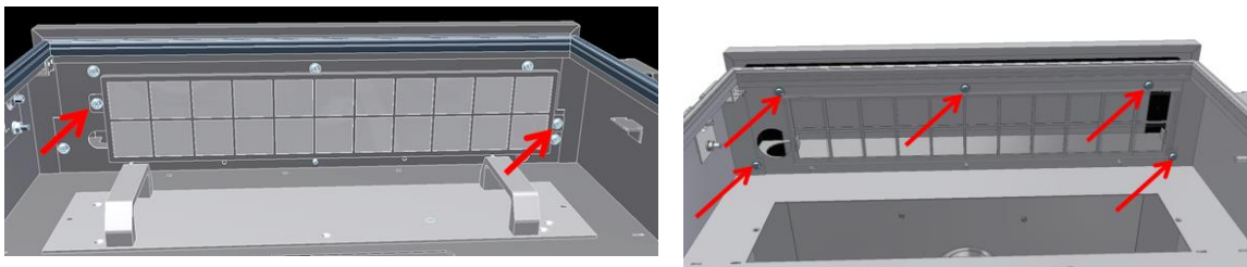
Abbildung 17: Luftfilter ausbauen (von vorne - unten)
