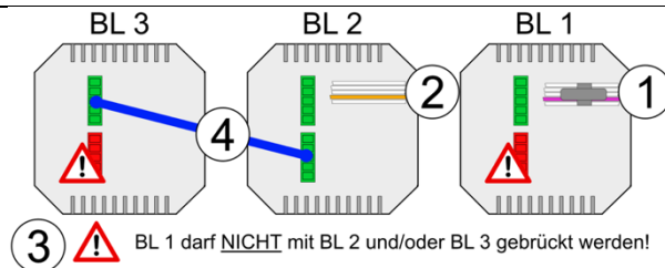
Abbildung 16: Batterielader 1, 2 und 3 Rückseite
