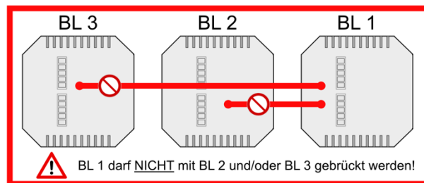
Abbildung 16: Batterielader 1, 2 und 3 Rückseite
