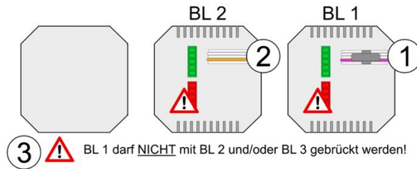
Abbildung 15: Batterielader 1 und 2 Rückseite
