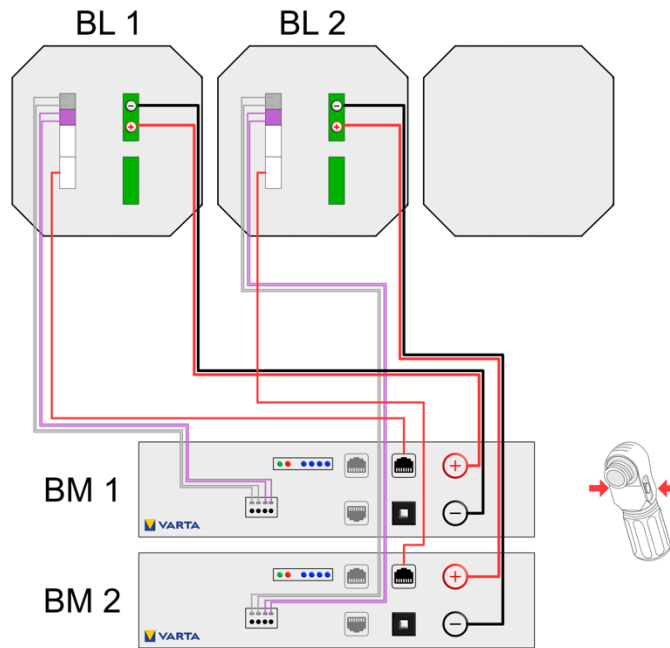
Abbildung 6: Batterielader 1 und 2, Batteriemodul 1 und 2
