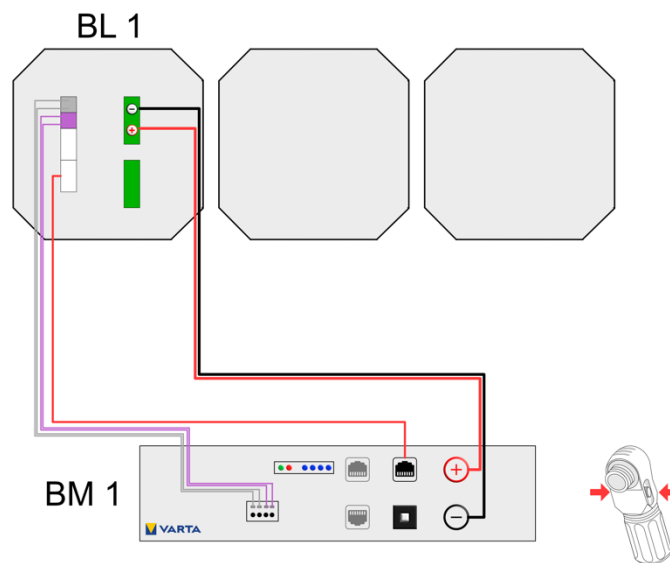
Abbildung 4: Batterielader 1 - Batteriemodul 1
