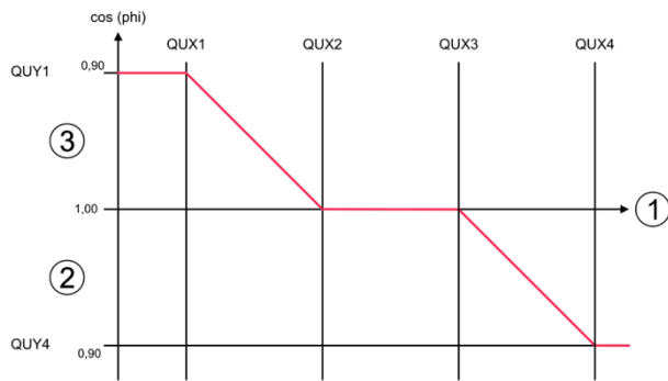
Abbildung 11: Q(U)-Kennlinie
