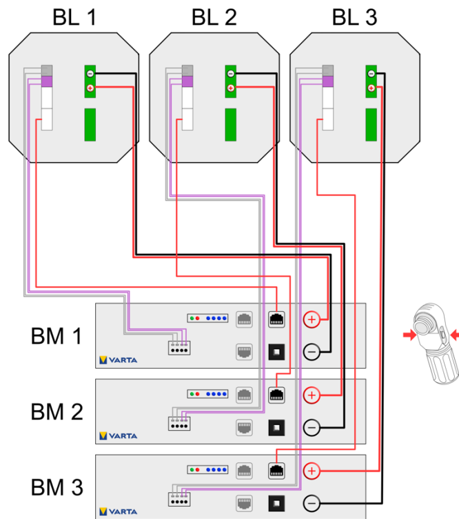
Abbildung 8: Batterielader 1 und 2, Batteriemodul 1, 2 und 3,
