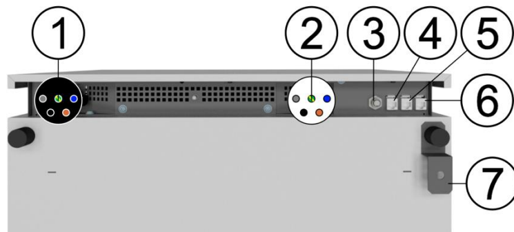
Abbildung 3: Rückseite Speicherschrank
