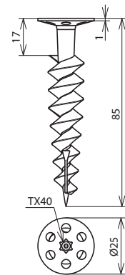
Maßbild HSPD HS4.5 L85 PA
