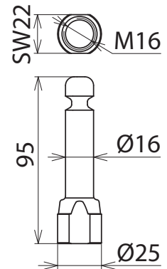
Maßbild EFP 16 RN M16
