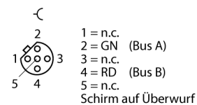
Anschlussbelegung links
