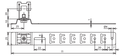
Maßbild DLH UG 8 H20 L475 CU
