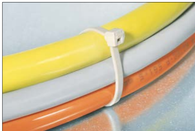
Der hitzebeständige PEEK-Kabelbinder PT220 für Hochtemperaturanwendungen.
