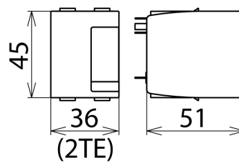
Maßbild DR MOD 4P 255 SN1871
