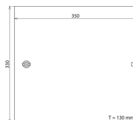
Maßbild DPG LSA 120 P
