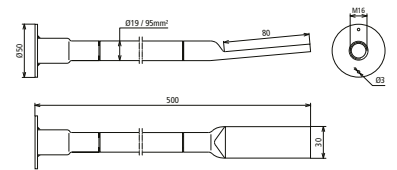
Maßbild D BEB 5 / EBS 15-03-19
