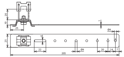
Maßbild DLH DG 8 H20 L205 V2A AL
