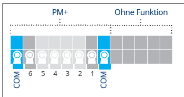
Abb.: PIN-Belegung an der Unterseite
