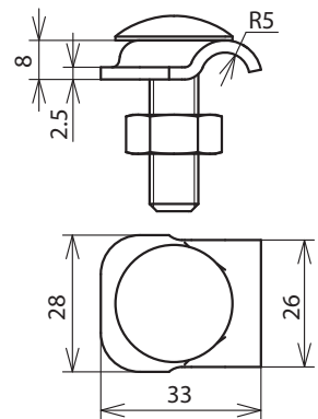
Maßbild KB 6.10 FRM10X35 STTZN
