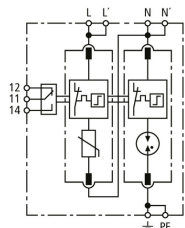
Principalschaltbild DG MP TT 2P 275 FM
