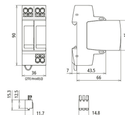
Maßbild DG MP TT 2P 275 FM
