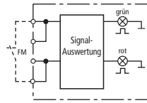
Prinzipschaltbild
