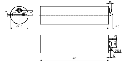
Maßbild
