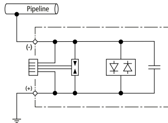
Prinzipschaltbild
