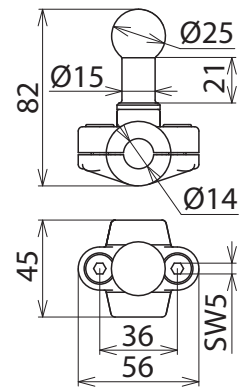
Maßbild KFP 25 RL 14
