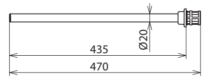
Maßbild S61 PS PHE 435
