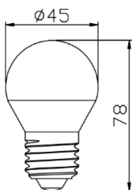
Abmessungsskizze LED MT65003
