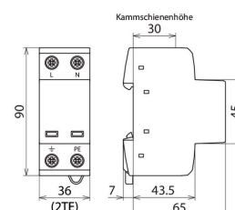
Maßbild DSH TT 2P 255
