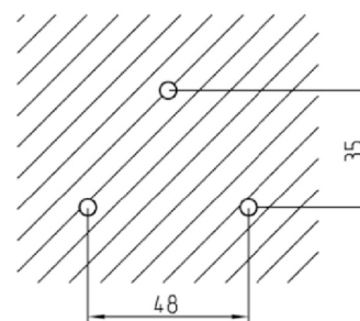
Bohrbild
