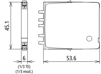
Maßbild BCO MOD ML2 BD EX 24
