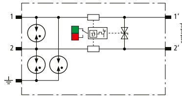
Prinzipialschaltbild BCO MOD ML2 BD EX 24
