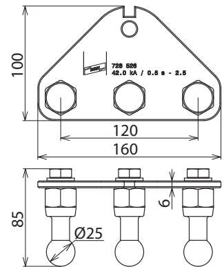
Maßbild EAPA 3 KFP 25 B13
