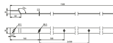
Maßbild AF 30X3.5 V4A ZW 1500
