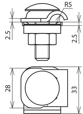
Maßbild MMVK 6.8 FRM10X35 CU
