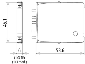
Maßbild BCO MOD ML2 BD 48
