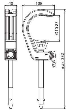
Maßbild
